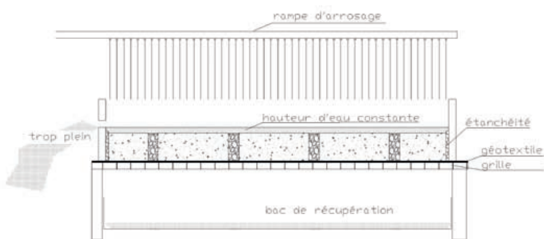
Schéma de l'essai de détermination du coefficient de perméabilité
