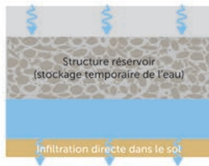
Figure 19 - Exemple de structure réservoir avec évacuation de l'eau par infiltration directe.
