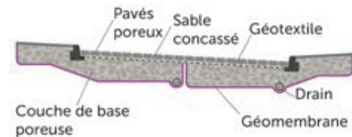
Figure 22 – Exemple de parking en pavés poreux.
