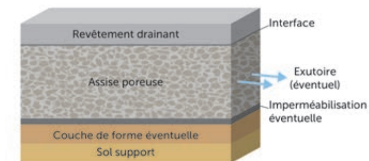
Figure 27 - Structure-type d'une voirie à assise poreuse et revêtement drainant.
